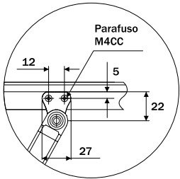
F0036NI - Placa para utilização em portas em perfil de alumínio largura 19/20mm
